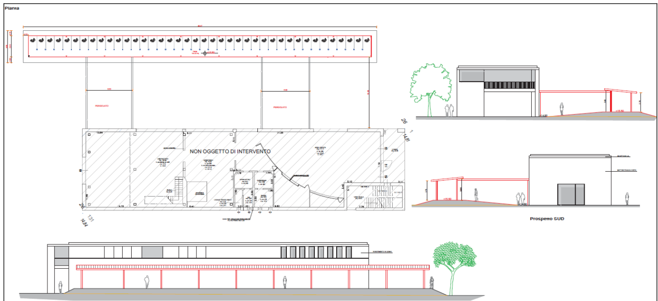
Progetto edilizio presentato – tav. 3 – PLANIMETRIA E PROSPETTI – stato comparato
