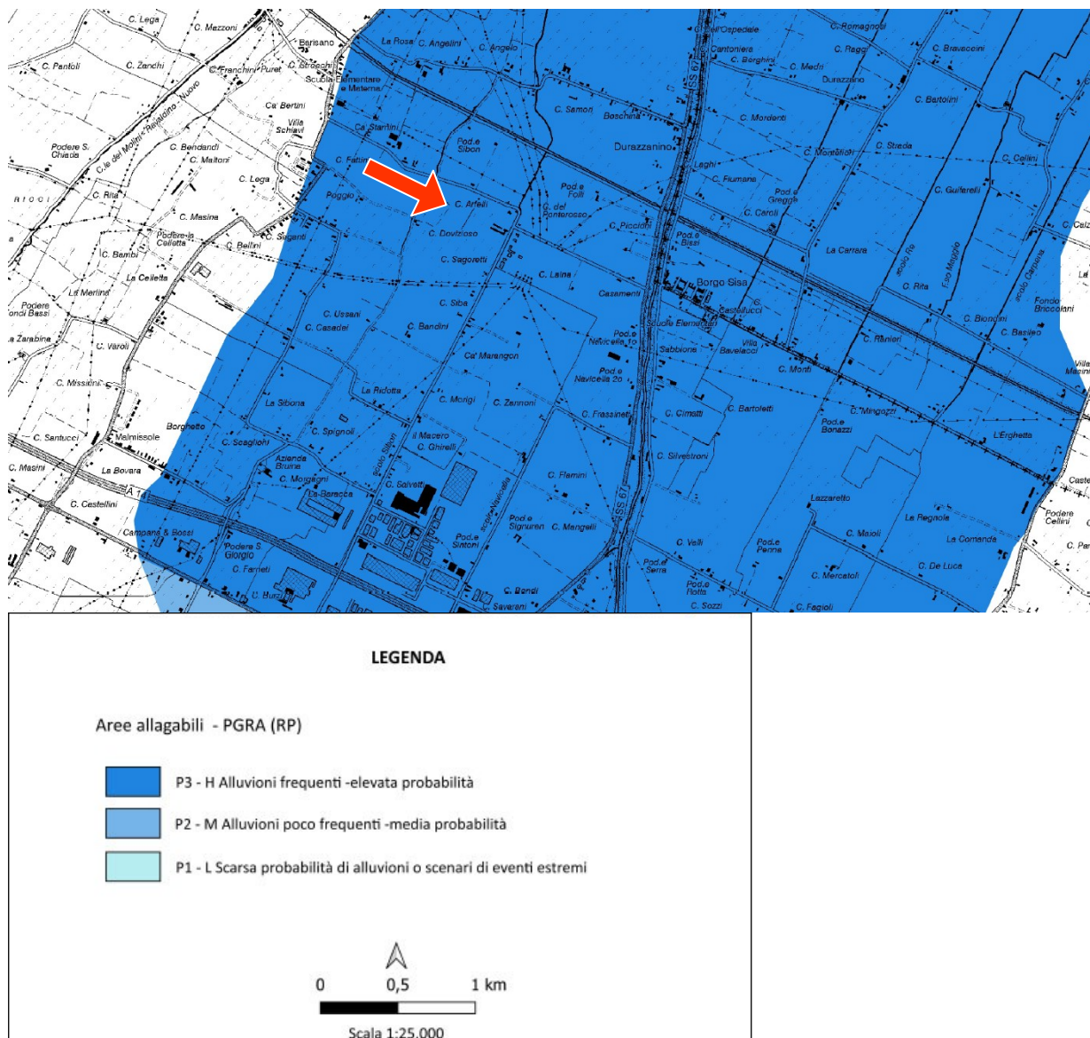
PROGETTO DI VARIANTE AL PAI PO – PGRA - AREE ALLAGABILI – Fiume Ronco (tav. 2)
